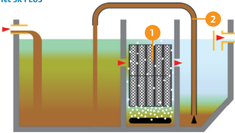
Schematische Darstellung der Funktionsweise einer belüfteten Festbetтанlage 3K PLUS®.
